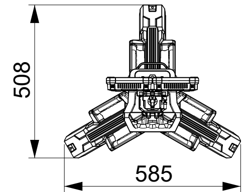
TL-200 Dual head Unit:mm
